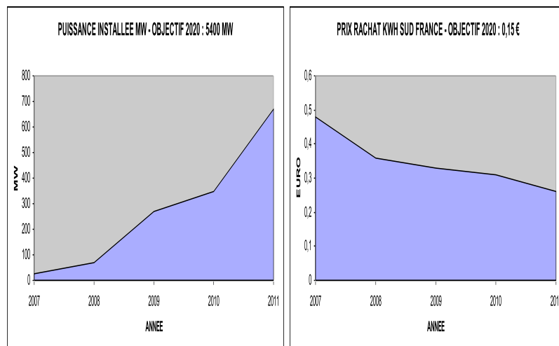
Graphique puissance installée fonction de l'année Graphique prix de rachat fonction de l'année
